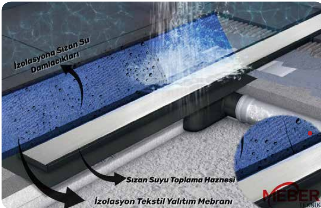
İzolasyona Kaçan Suyu Toplama Haznesi
